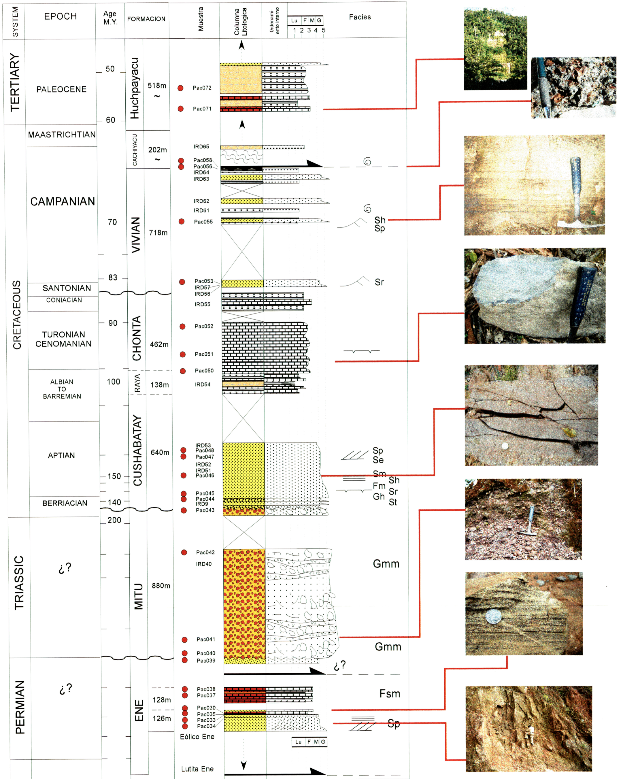
Anexo 6.- Columna estratigráfica de los afloramientos de San Matías con sus correspondientes datos de campo de IRD 1995 y IRD 2006 (puntos rojos).
