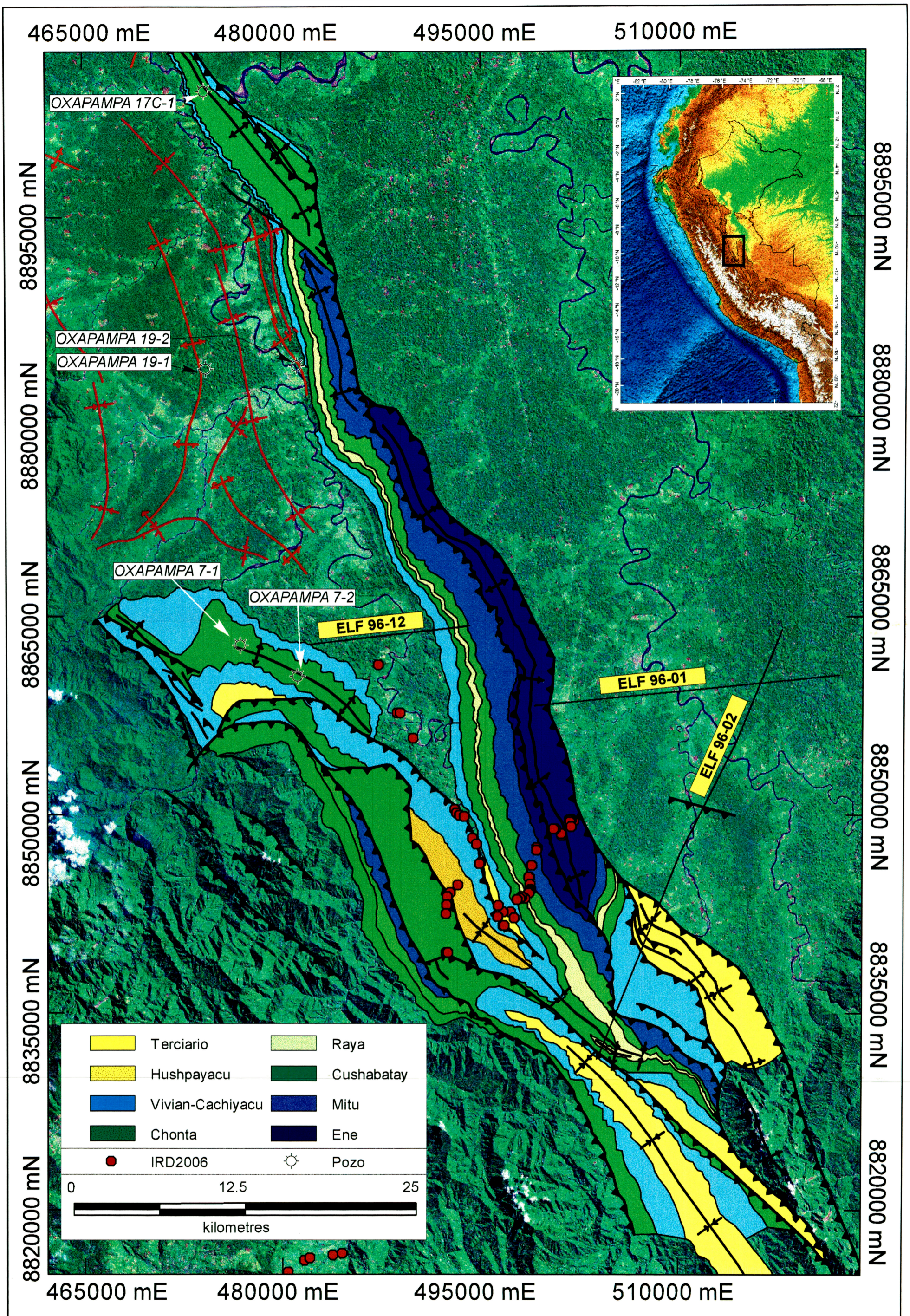
Anexo 7.- Mapa geológico final de la Sub. Cuenca Pachitea, elaborado a partir de datos de IRD1995, 2006 e información de campañas de campo anteriores (PANENERGY, OXY y ELF).
