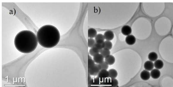
Figura 9. Imágenes obtenidas por microscopía electrónica de transmisión correspondientes a las partículas de poliestireno de a) 1,03 \mu\text{m} y b) 0,49 \mu\text{m} .
