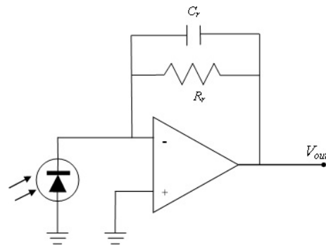
Figura 3. Fotodiodo conectado en modo fotovoltaico a un amplificador operacional como convertidor corriente-voltaje. La fotocorriente genera una caída de potencial en la resistencia R_f , esta caída de potencial es igual al voltaje de salida del amplificador operacional. El condensador C_f es utilizado para eliminar oscilaciones debido a capacitancias parásitas a la salida del circuito.
