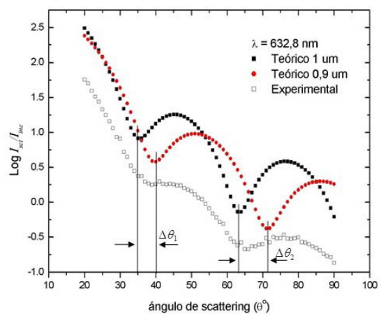
Figura 10. Comparación entre la curva experimental de las microesferas de 1,03 \mu\text{m} de diámetro nominal y dos curvas teóricas para microesferas de 0,9 y 1 \mu\text{m} de diámetro. Las posiciones angulares de los mínimos de la curva experimental se encuentran en los intervalos \Delta\theta generados por estas curvas teóricas, \Delta\theta_1 \approx 5^\circ y \Delta\theta_2 \approx 7^\circ
