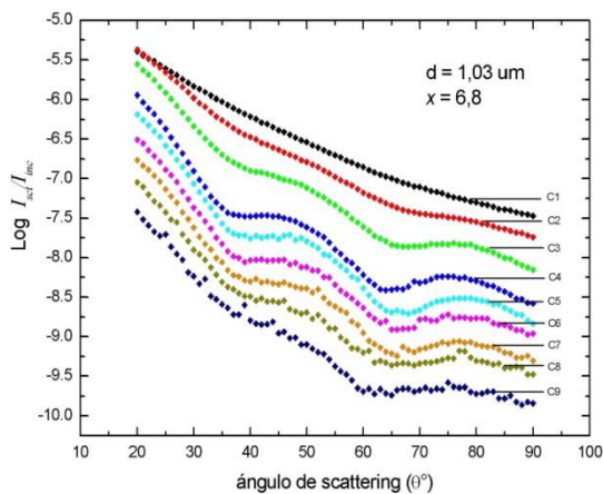
Figura 8. Curvas de scattering experimentales para muestras de diferentes concentraciones correspondientes a las partículas de poliestireno de 1,03 \mu\text{m} diámetro y longitud de onda de 632,8 nm. Se muestran curvas para nueve concentraciones diferentes, donde C1 > C2 > C3 > C4 > C5 > C6 > C7 > C8 > C9 ; con C4 \sim 10^6 partículas/ml.
