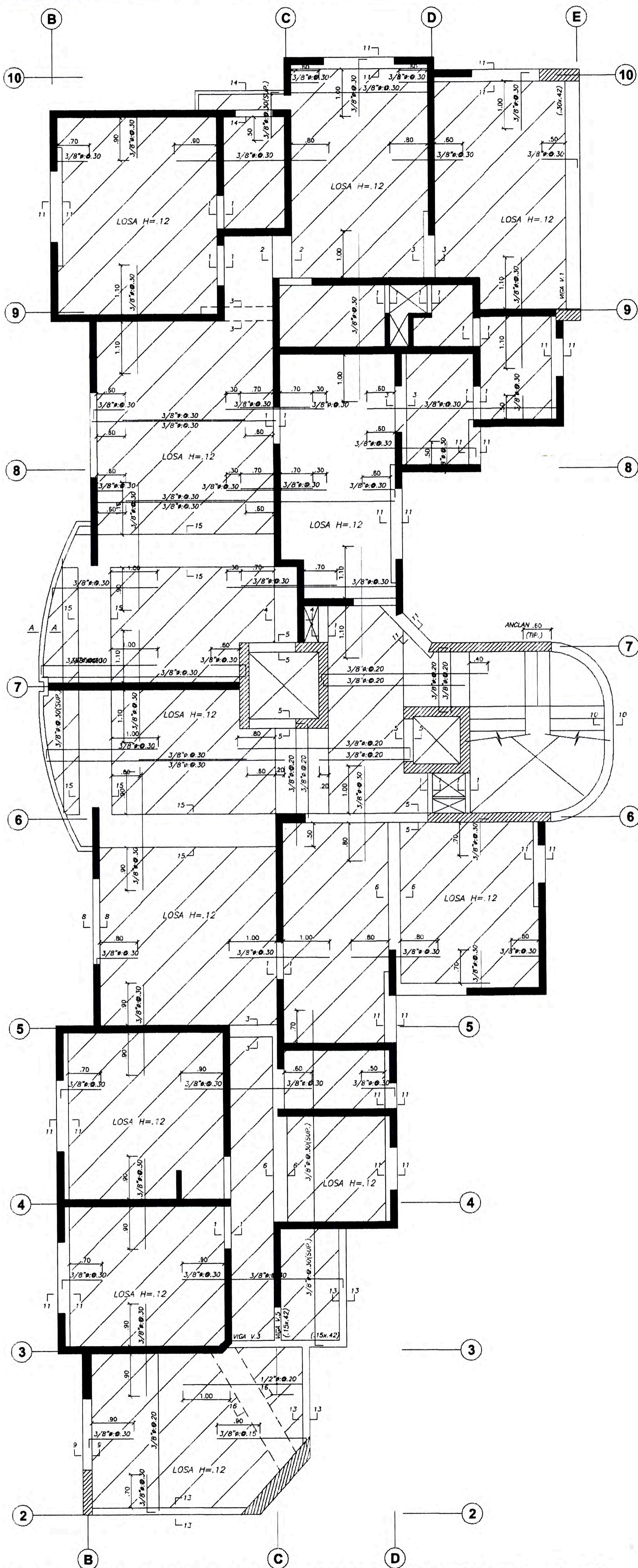
iii) PLANTA TIPICA DE LOSA- ESTRUCTURAS. E-03
