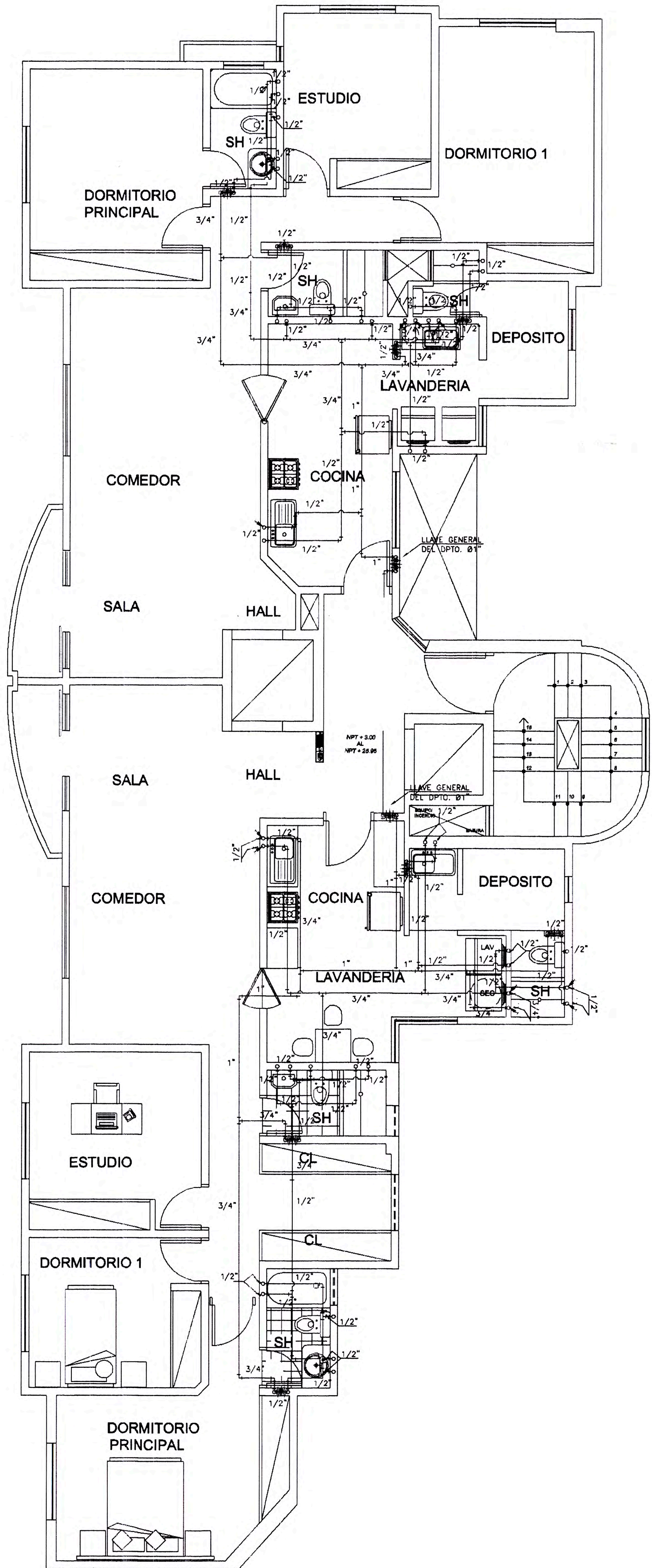
PLANTA TIPICA
