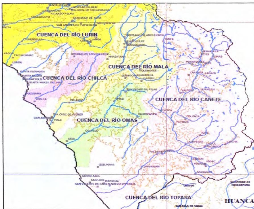
FIGURA N°1.02 CUENCAS DE LA PROVINCIA DE CAÑETE
