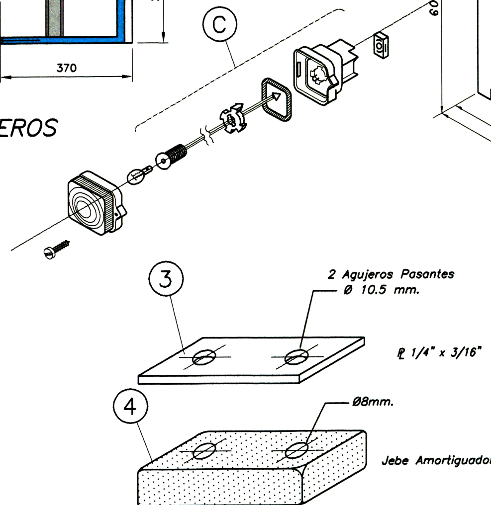
VISTA POSTERIOR
