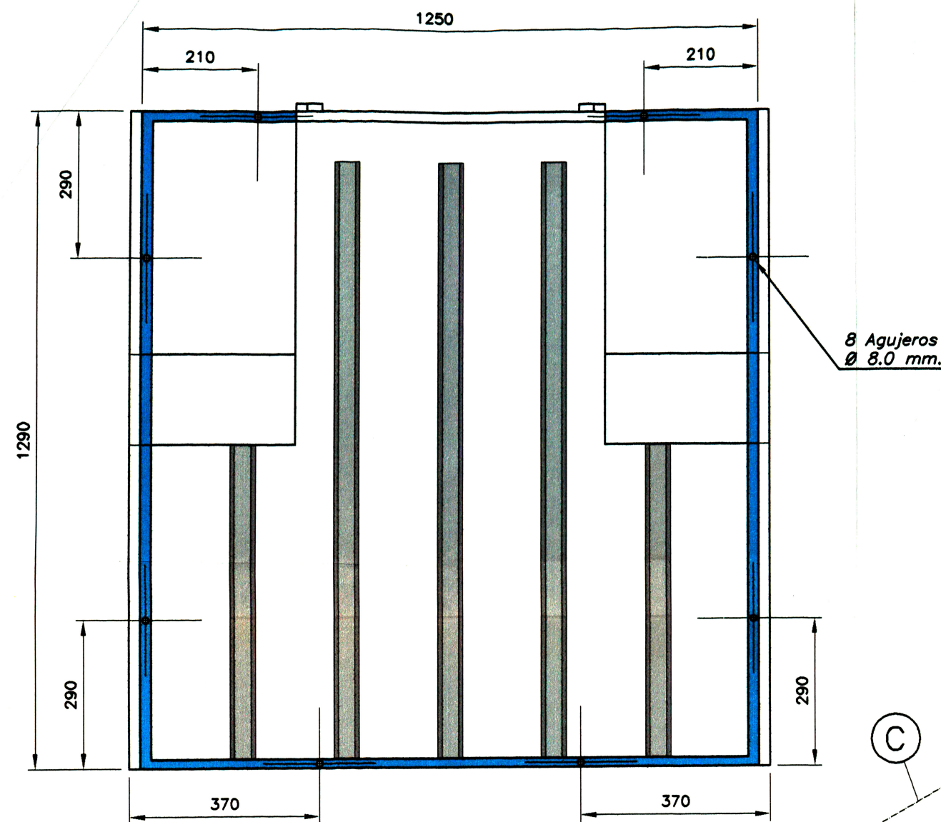
POSICION DE AGUJEROS DE ENSAMBLE
