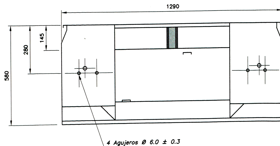
VISTA POSTERIOR
